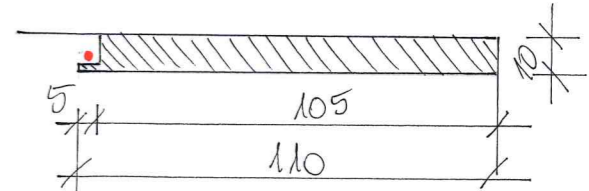
3p. XIII. Pozsonyi utca - Nappali almelezet M=1:50
